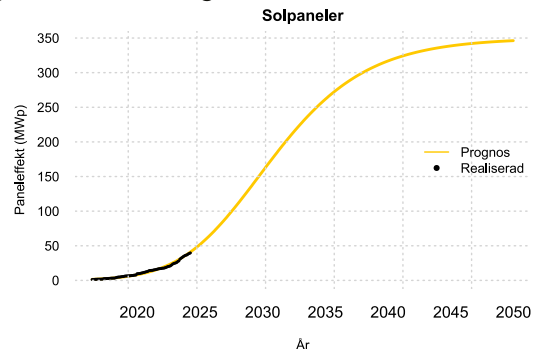
Bild 10. Kumulativ nominell effekt och prognos för installerade solpaneler.
